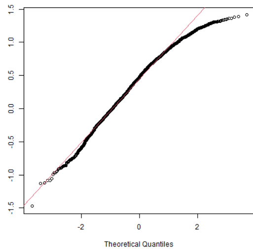
(d) Female QQ-plot
