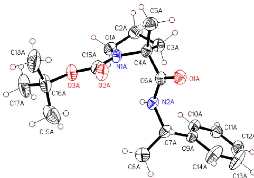
22g ( R,S )
